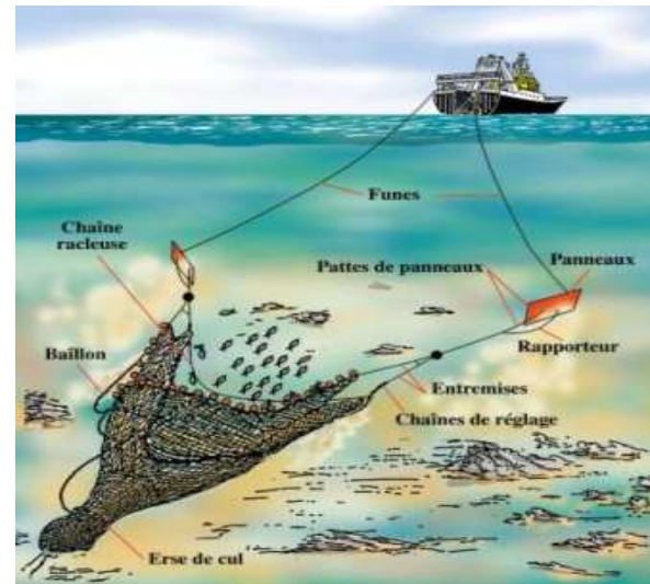
LE CHALUT DE FOND
